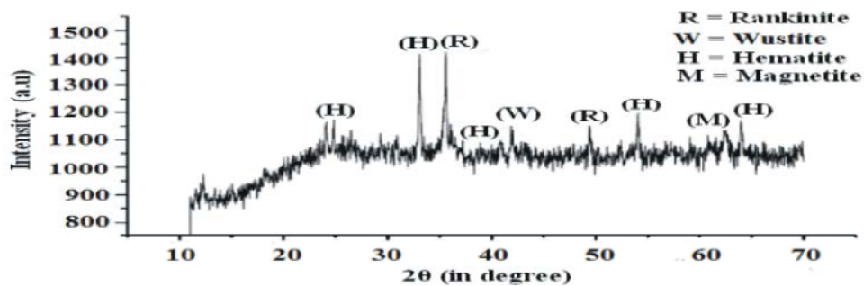
Fig. 5: XRD of SMS slag
